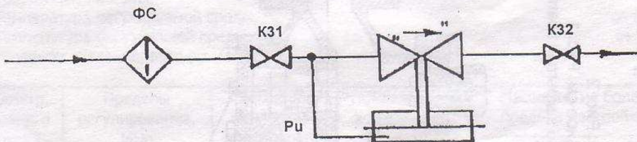
Б) регулирование давления "до себя"
