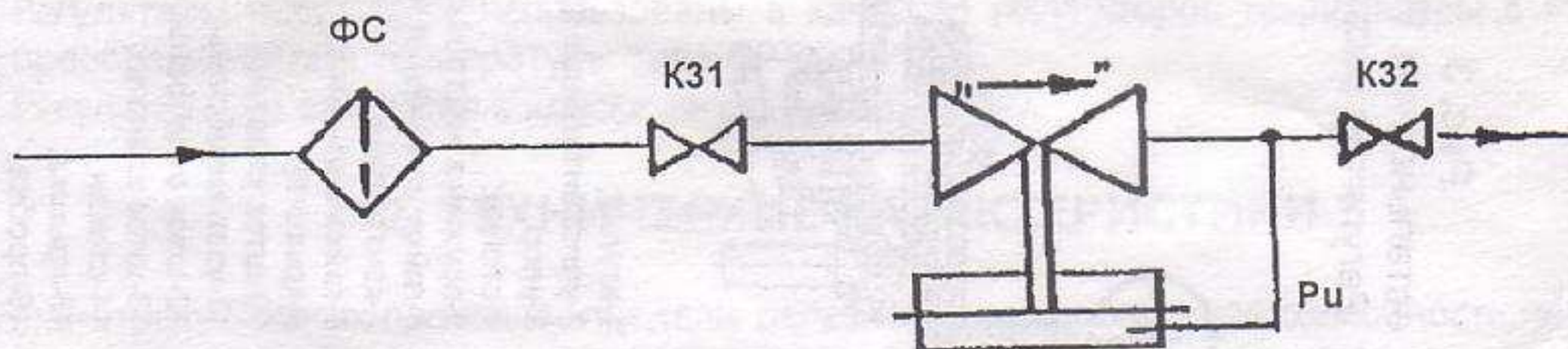
А) регулирование давления "после себя"
