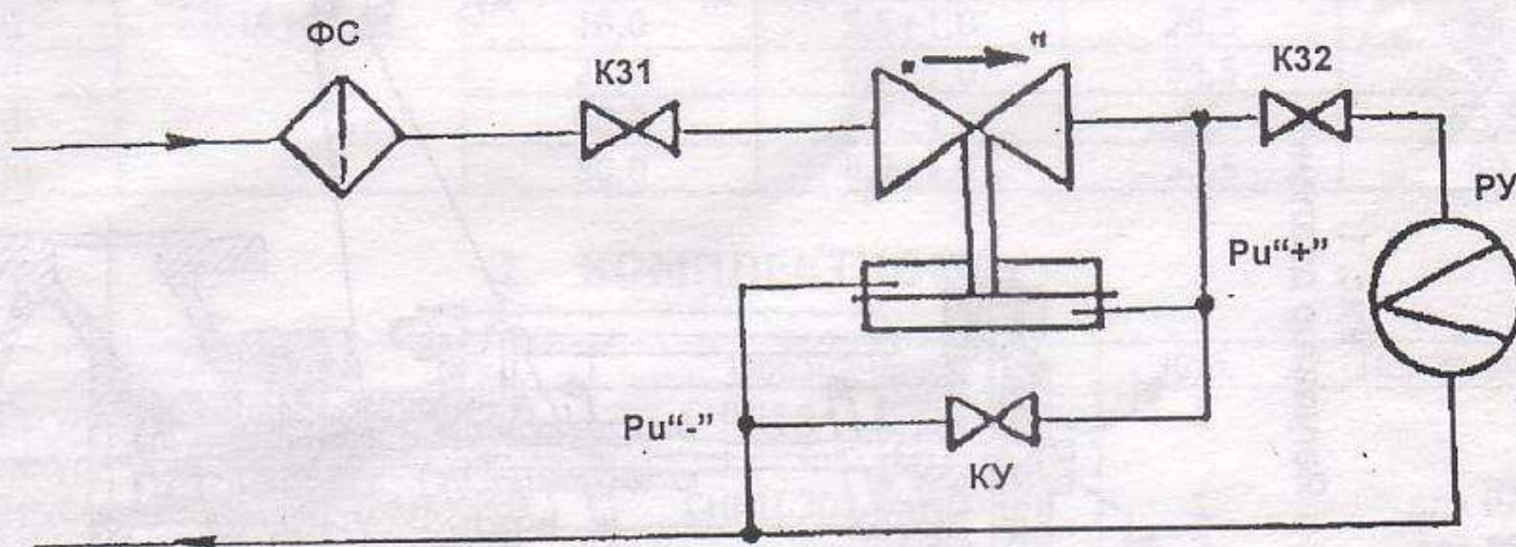
В) регулирование расхода (перепада давлений)
