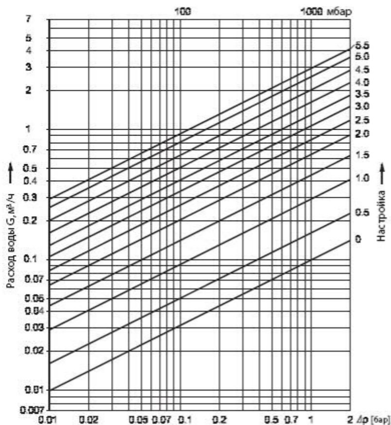
Расходная характеристика
