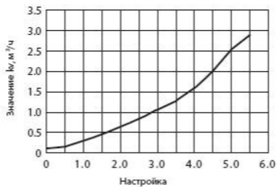
Расходная характеристика
