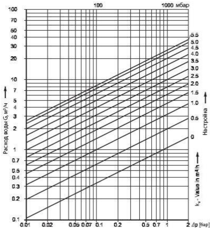
Расходная характеристика
