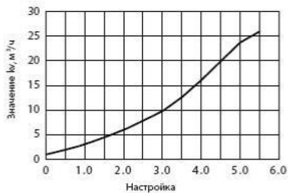
Расходная характеристика
